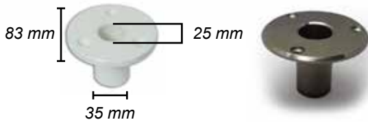
SL12049 | Pasarella Montaj Yuvası Plastik SL12050 | Pasarella Montaj Yuvası CR-NI Ø 25mm
