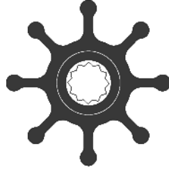
SL48112 | Impeller Lastığı Sealux Çap: 65mm Genişlik: 50,8mm Kanat Sayısı: 8 Jabsco Kod: 920-0001 920-0003
