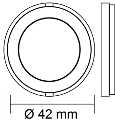
SL16902 | Merdiven Lambası BEYAZ LED 12V SL16902-M | Merdiven Lambası MAVİ LED 12V
