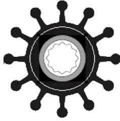
SL48101 | Impeller Lastığı Sealux Çap: 57mm Genişlik: 31,5mm Kanat Sayısı: 12 Jabsco Kod: 1210-0001 1210-0003
