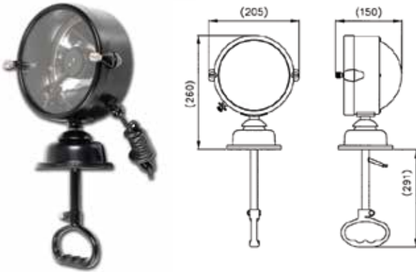
SL18101 | Aldis El Mors Feneri
