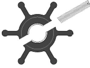
SL48123 | Impeller Lastığı Sealux Çap: 51mm Genişlik: 22mm Kanat Sayısı: 6 Jabsco Kod: 653-0001
