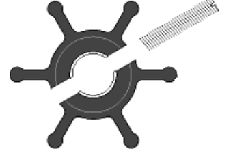
SL48110 | Impeller Lastığı Sealux Çap: 51mm Genişlik: 22mm Kanat Sayısı: 6 Jabsco Kod: 673-0001 673-0003
