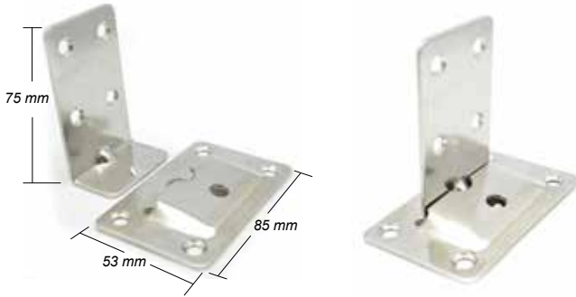
SL40030 | Geçme Ayak CR-NI 90
