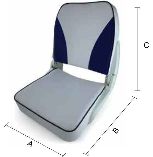
SL28055 | Katlanır Koltuk Beyaz+Lacivert A: 45cm B: 36cm C: 48cm
