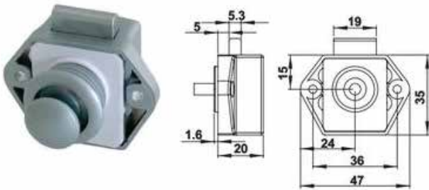
SL 40050 | Basmalı Dolap Kulbu Gri Aks Mesafesi : 15 mm Çap : 20 mm
