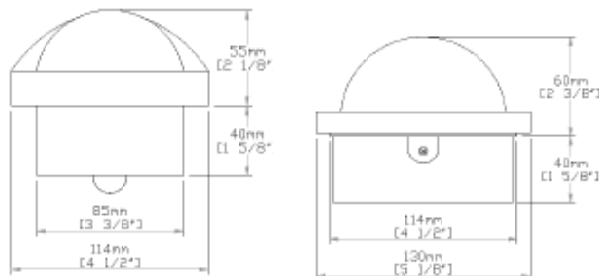
SL53914 | Pusula Autonautic C15-063 Siyah
